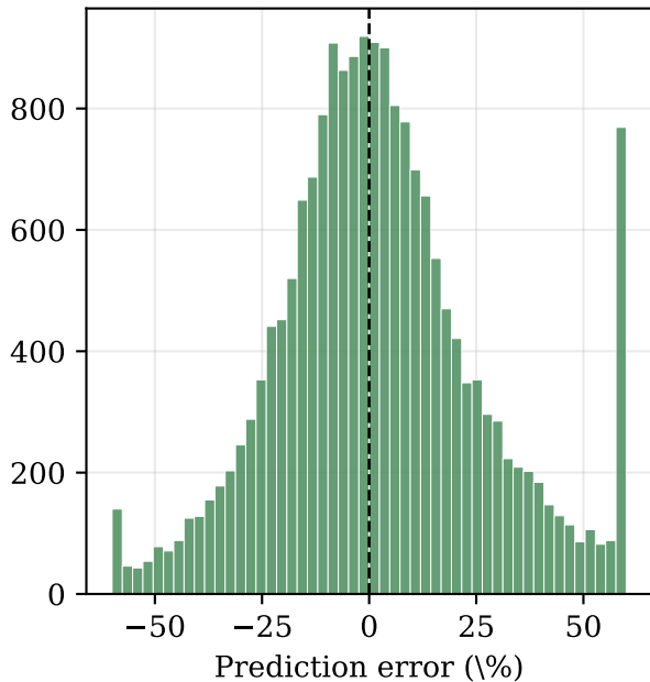
Errors (median |\cdot|=14.0\% )
